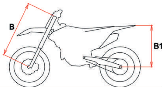
Рисунок 5.34. Замеры в разгрузке.
