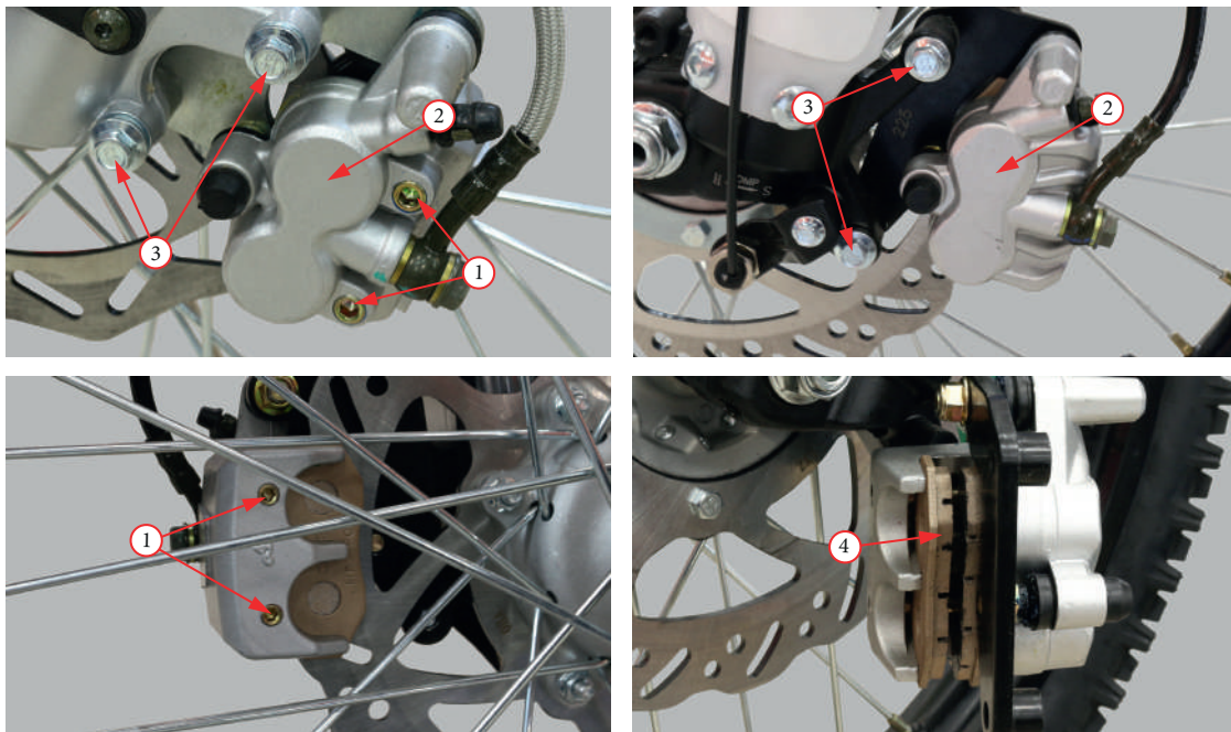
Фото 5.24. Замена передних тормозных колодок.
