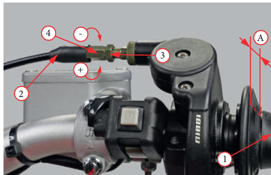
Фото 5.9. Регулировка свободного хода рукоятки акселератора.
