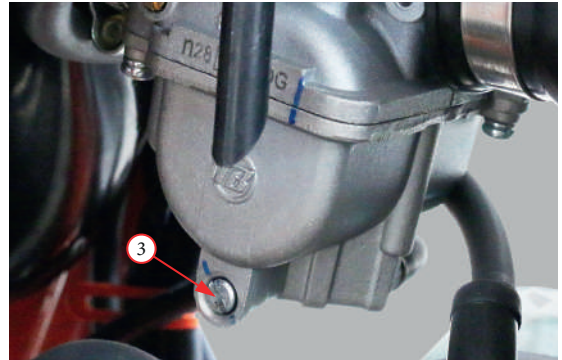
Фото 5.10. Регулировка холостых оборотов.
