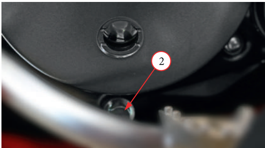
Фото 5.3.1. Сливной болт в двигателе LX1E66MM (MT-250 2T).
