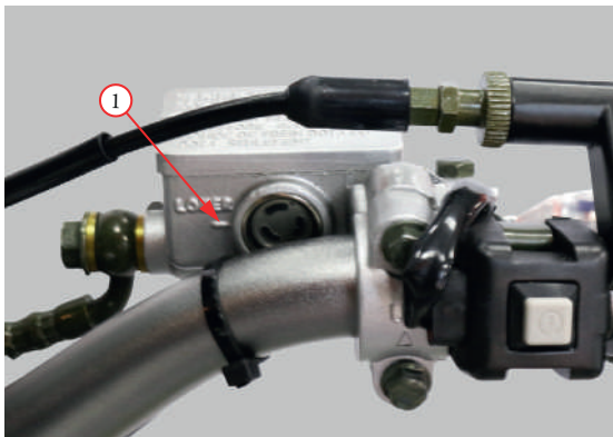
Фото 5.19. Проверка уровня тормозной жидкости.
