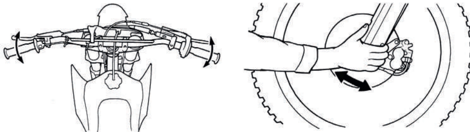
Рисунок 5.32. Проверка рулевой колонки.
