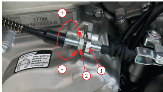
Фото 5.13. Регулировка сцепления на двигателе.
