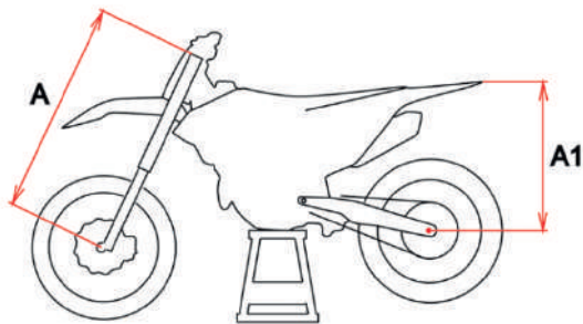
Рисунок 5.33. Замеры на подставке.
