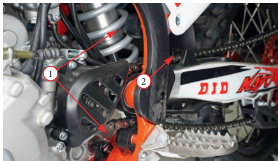
Фото 5.28. Ролики цепи – 1, слайдер-успокоитель – 2.
