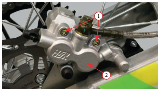
Фото 5.25. Замена задних тормозных колодок.
