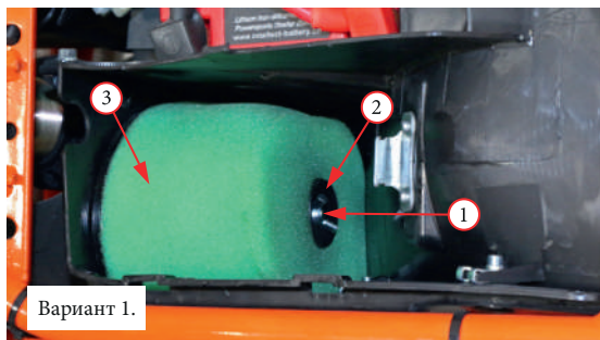
Фото 5.7. Варианты исполнения воздушных фильтров.
