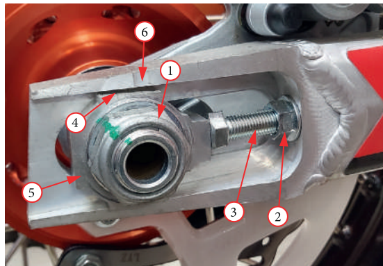
Фото 5.29. Регулировка натяжения цепи.
