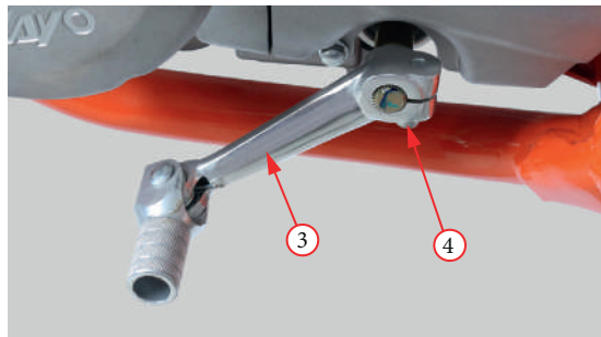
Фото 5.14. Регулировка положения рычага передач.
