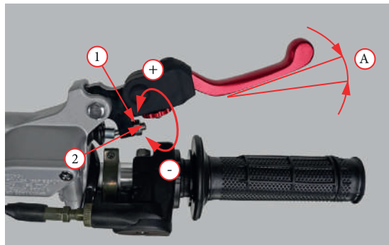
Фото 5.17. Регулировка передних тормозов.
