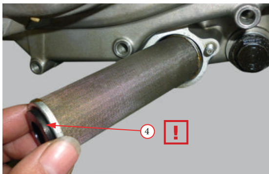
Фото 5.4. Замена масла в двигателях с масляным фильтром.
