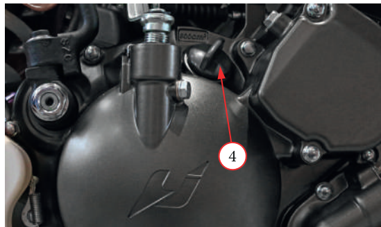
Фото 5.1.1. Исполнение смотрового окна и крышки горловины двигателей LX1E66MM (MT-250 2T).
