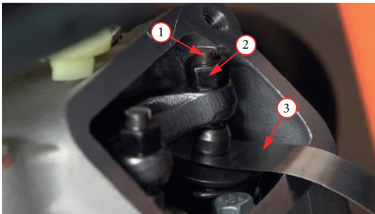
Фото 5.40. Регулировка теплового зазора: 1 – регулировочный винт; 2 – контргайка; 3 – щуп.
