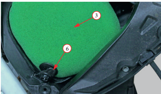
Фото 5.8. Элементы воздушного фильтра.
