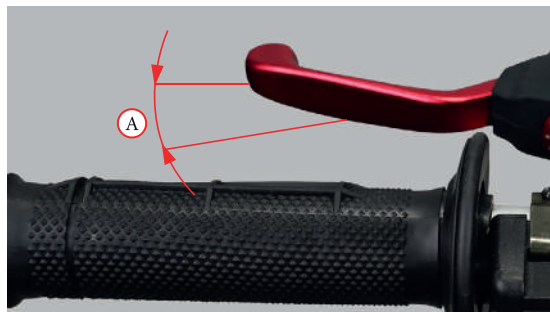
Фото 5.11. Свободный хода рычага – А.
