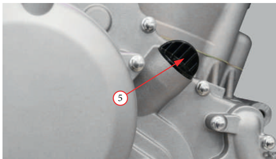
Фото 5.4.1. Замена масла в двигателях с масляным фильтром.
