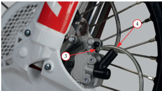
Фото 5.23. Прокачка тормозной системы.
