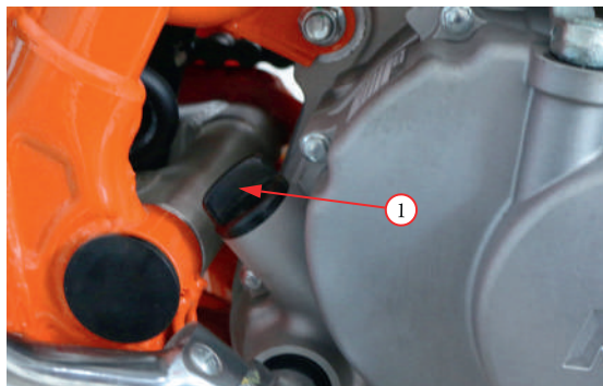
Фото 5.5. Замена масла в двигателях YX166FMM, ZS169FMM и ZS172FMM.
