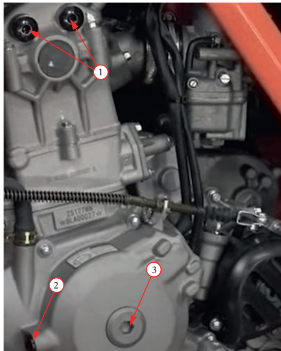
Фото 5.36. Крышки окон левой стороны двигателя: 1 – окна с метками «L» (левое) и «R» (правое); 2 – боковое смотровое окно; 3 – окно к валу.
