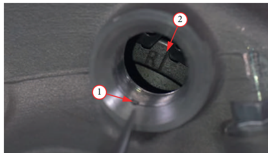
Фото 5.38. Совмещение риски 1 на боковом окне с меткой 2 на валу.
