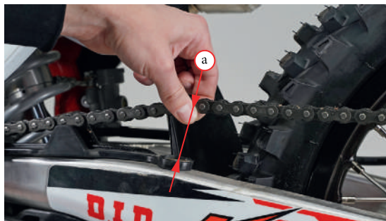
Фото 5.26. Замер провисания цепи.
