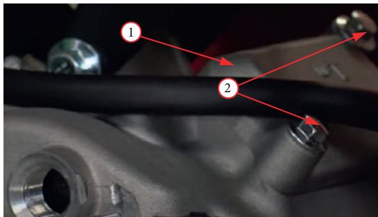
Фото 5.35. Снятие крышек клапанов: 1 – крышка впускного клапана; 2 – болты крепления крышки.
