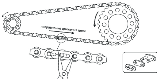
Рисунок 5.31. Установка элементов замка цепи.
