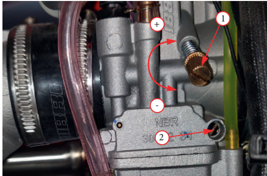
Фото 5.10. Регулировка холостых оборотов.
