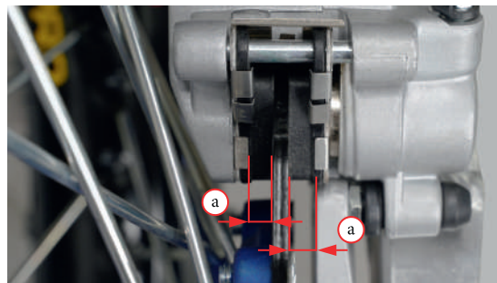
Фото 5.21. Контроль тормозных колодок.
