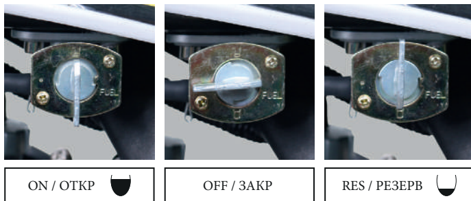
Фото 3.1. Положения крана подачи топлива.
