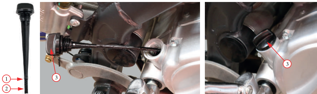
Фото 5.3. Указатель уровня масла в двигателях.
