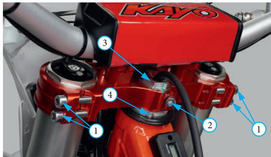
Фото 5.34. Регулировка подшипников рулевой колонки модели Kayo K6.
