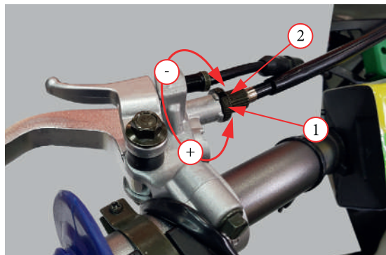
Фото 5.12. Регулировка свободного хода рычага сцепления.
