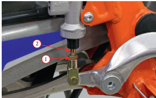
Фото 5.18. Регулировка высоты педали тормоза.
