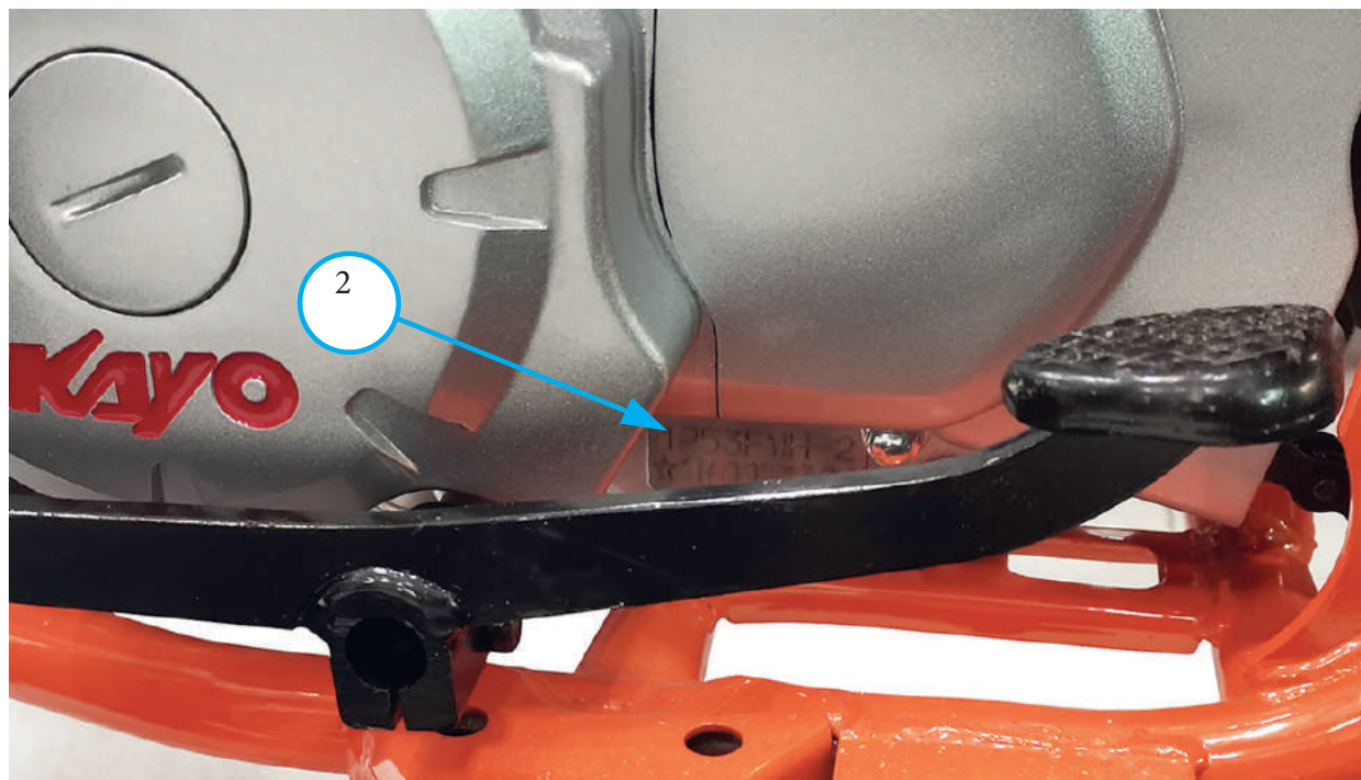
Фото 1.3. Место расположения серийного номера двигателя - 2
