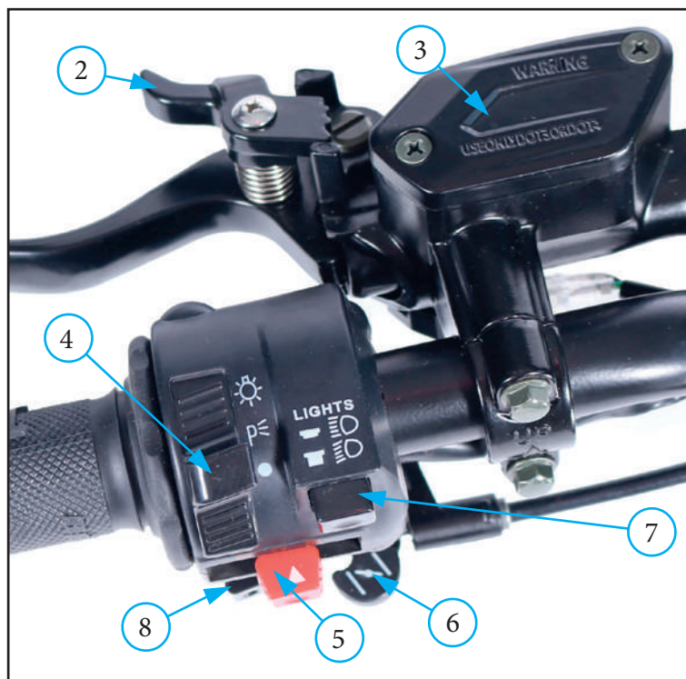
Фото 2.6. Переключатели левого блока комплекта запчастей:
