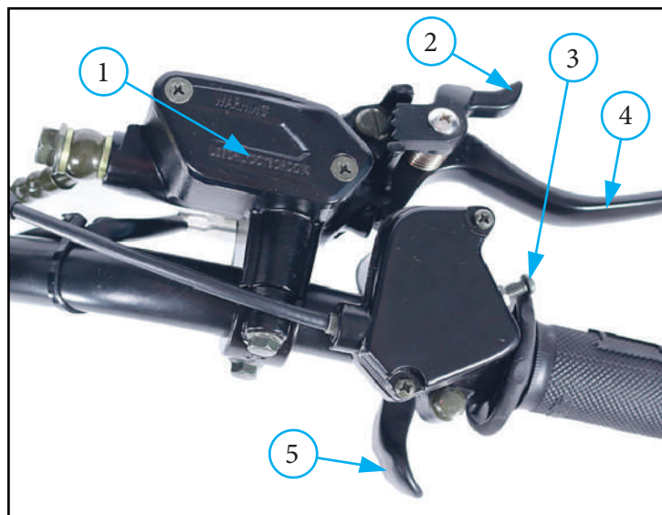
Фото 2.5. Переключатели правого рулевого блока комплекта запчастей: 1 - бачок переднего тормоза; 2 - фиксатор парковочного тормоза; 3 - регулятор ограничения акселератора; 4 - рычаг переднего тормоза; 5 - рычаг акселератора
