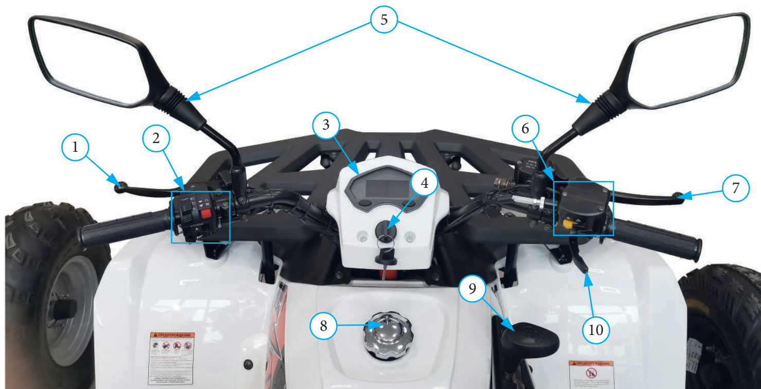
Фото 2.2.1 Приборы и органы управления квадрицикла: 1 – рычаг сцепления; 2 – левый рулевой блок; 3 – приборная панель; 4 – замок с ключом зажигания; 5 – зеркала заднего вида; 6 – правый рулевой блок; 7 – ручка переднего тормоза; 8 – крышка топливного бака; 9 – рычаг переключения передач; 10 – рычаг акселератора
