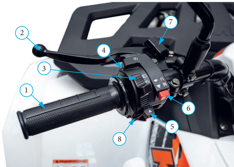
Фото 2.8. Переключатели левого блока квадрицикла: 1 – левая ручка; 2 – стояночный тормоз; 3 – переключатель фары (выключено/ближний/ дальний); 4 – кнопка электростартера; 5 – включатель указателей поворота; 6 – кнопка включения питания; 7 – фиксатор стояночного тормоза; 8 – кнопка звукового сигнала
