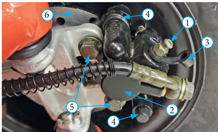
Фото 5.12. Тормозной узел:
